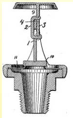
1890: Головка спринклера с использованием частей, сваренных вместе с помощью легкоплавкого сплава Вуда и механизма рычажного усилия (патент Фредерика Гриннеля N°432403)
